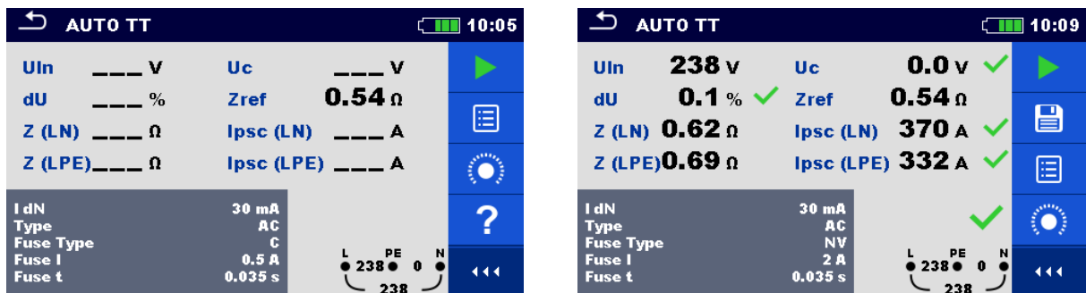
Рисунок 8.5: Примеры с результатов измерения АВТО ТТ.
