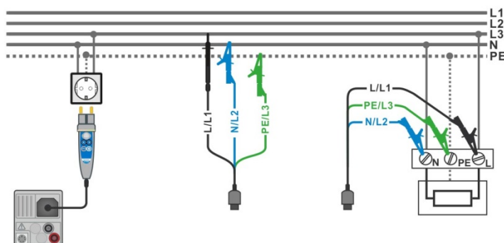
Рисунок 7.3: Подключение щупа «commander» с вилкой и 3-проводного измерительного кабеля в однофазной системе.
