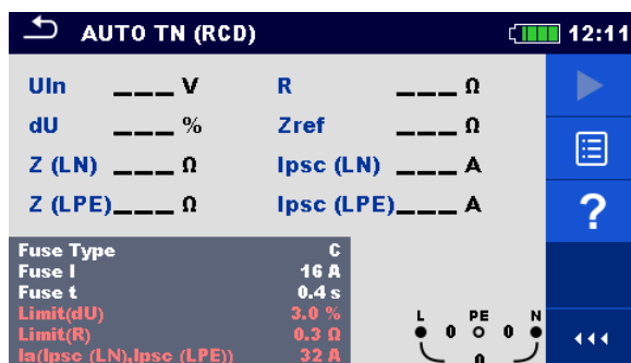
Рисунок 8.6: Меню АВТО TN (УЗО).
