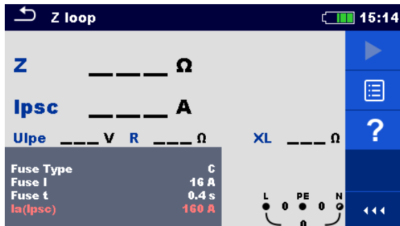
Рисунок 7.28: Меню Z конт.
