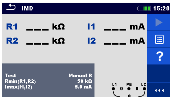
Рисунок 7.71: Меню IMD (устройств контроля изоляции).
