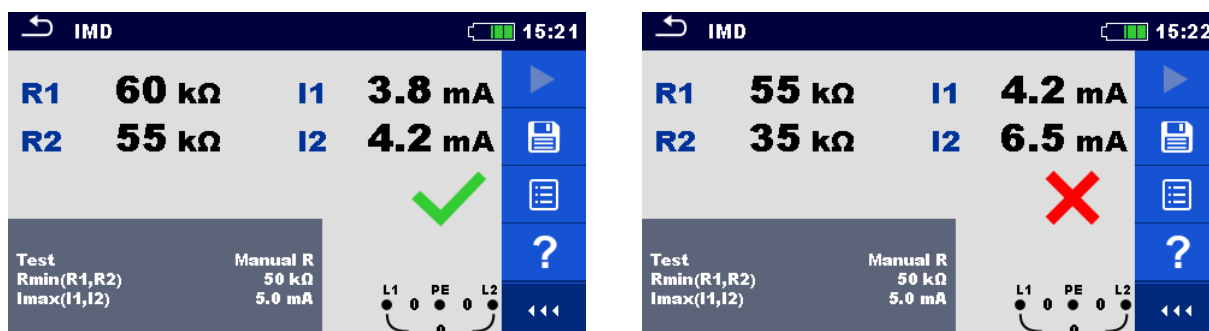
Рисунок 7.73: Пример результатов испытания IMD (устройства контроля изоляции).
