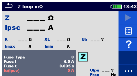
Рисунок 7.34: Меню Z конт мΩ (сопротивление контура Z, мОм).
