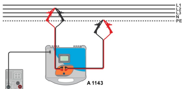
Рисунок 7.35: Высокоточное измерение полного сопротивления контура с помощью адаптера A 1143.
