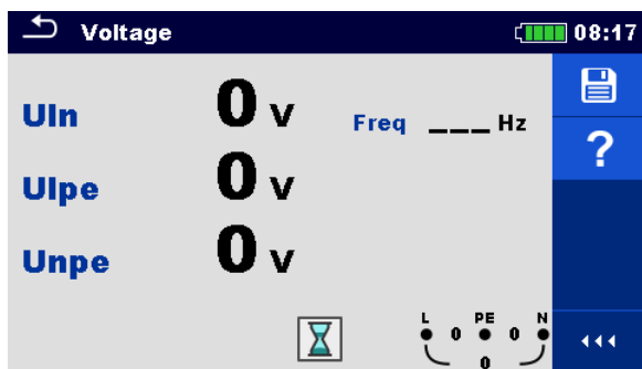
Рисунок 7.1: Меню измерения напряжения
