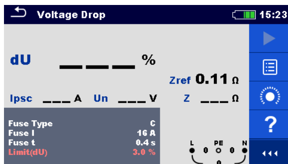
Рисунок 7.46: Пример результатов измерения Zоп (шаг 1).
