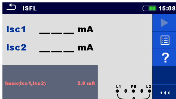
Рисунок 7.67: Меню ISFL (тока утечки первичного повреждения).
