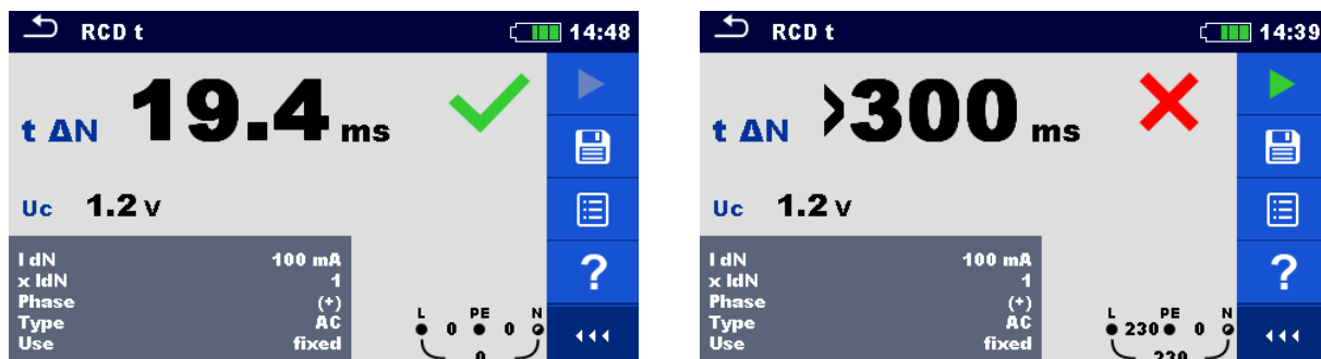
Рисунок 7.25: Пример результатов измерения времени срабатывания.
