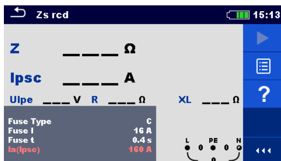
Рисунок 7.31: Меню Z_s УЗО.
