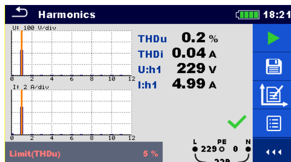
Рисунок 6.5: Пример результатов измерения гармоник.
