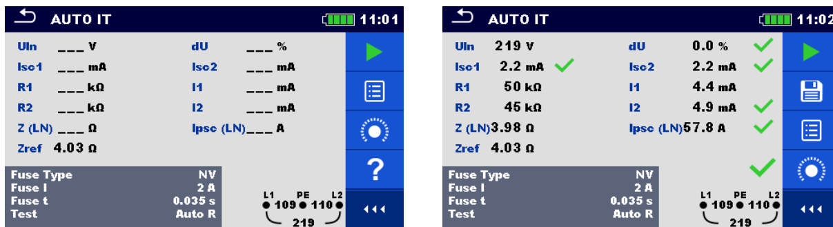
Рисунок 8.14: Примеры с результатов измерения AUTO IT.
