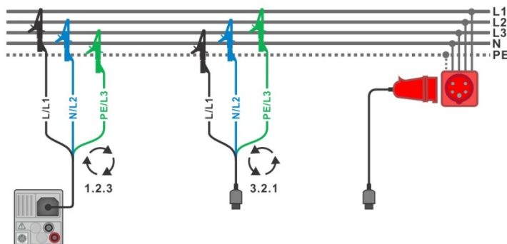
Рисунок 7.2: Подключение 3-проводного измерительного кабеля и опционального 3-фазного адаптера в трехфазной системе.
