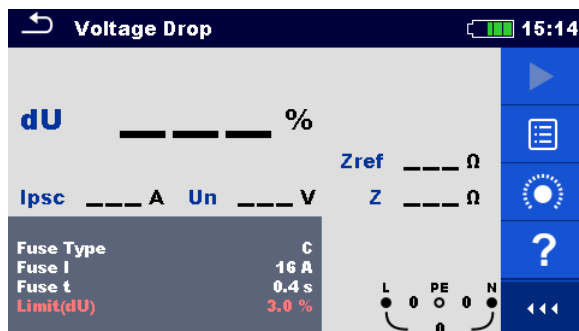
Рисунок 7.44: Меню падения напряжения.
