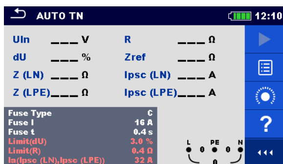
Рисунок 8.9: Меню АВТО TN.
