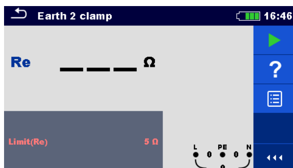
Рисунок 7.52: Меню Заземление (клещи).
