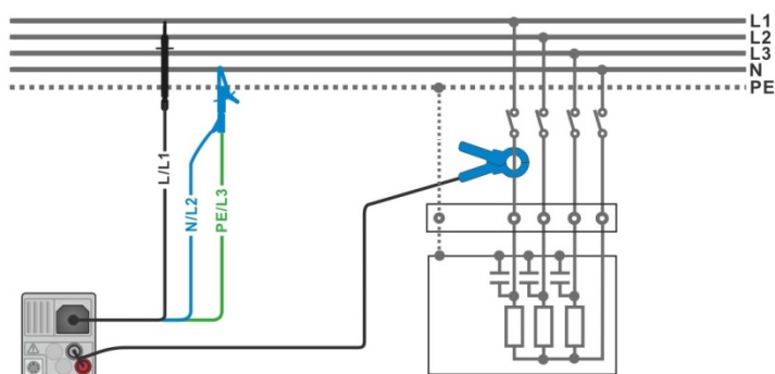
Рисунок 7.59: Измерение мощности.
