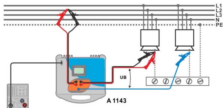
Рисунок 7.36: Измерение контактного напряжения с помощью адаптера А 1143.
