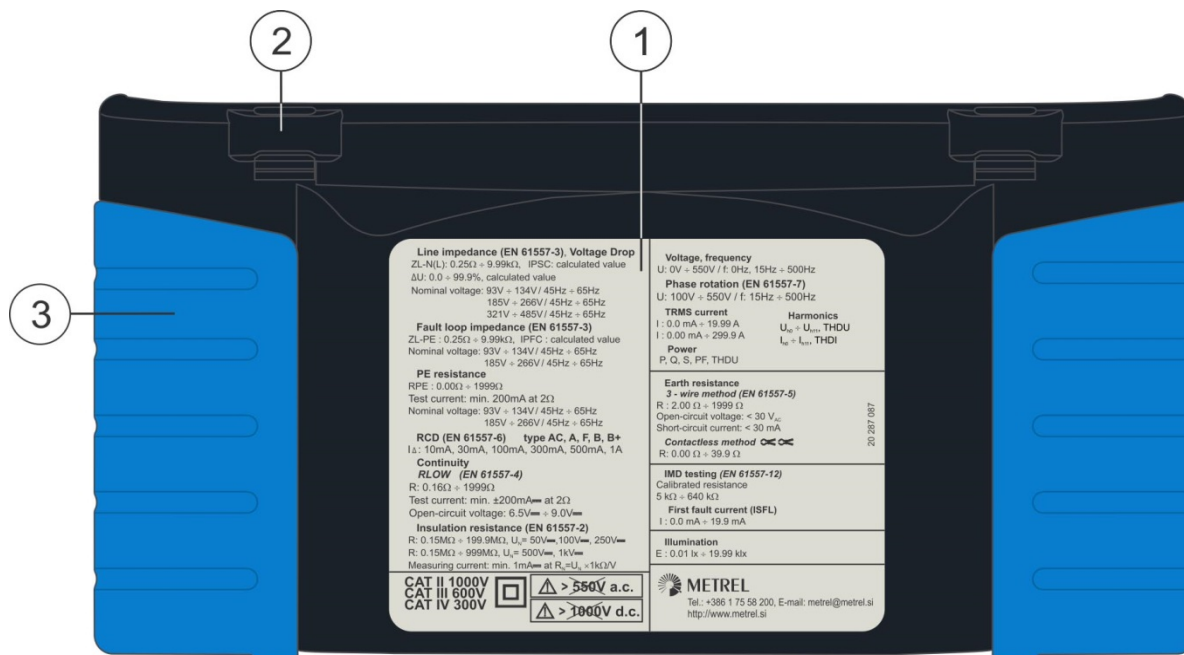
Рисунок 3.5: Вид снизу
