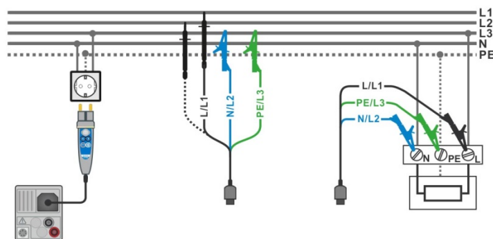
Рисунок 7.39: Подключение щупа «commander» с вилкой или 3-проводного измерительного кабеля при измерении полного сопротивления линии (фаза-нейтраль или фаза-фаза).
