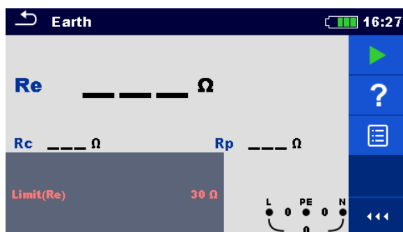
Рисунок 7.48: Меню заземления.
