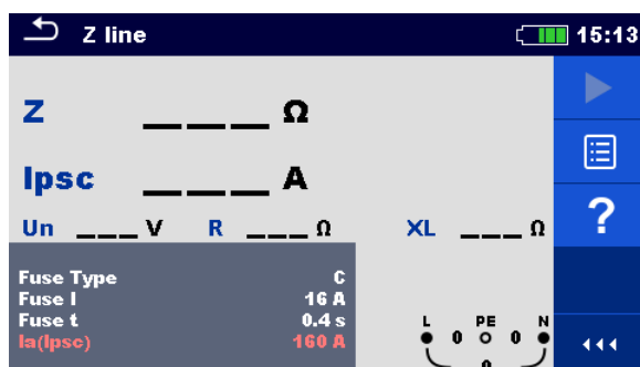
Рисунок 7.38: Меню измерения Z лин.
