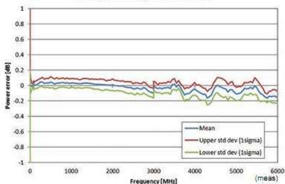
Частотная характеристика
