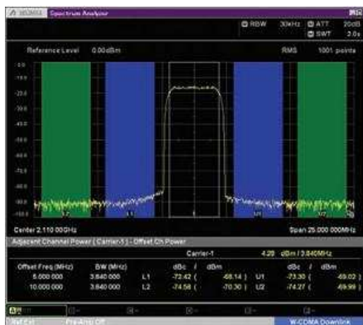
Коэффициент утечки по соседнему каналу W-CDMA (1 несущая) Шаблон формы волны (TestModel1, 64DPCH)
