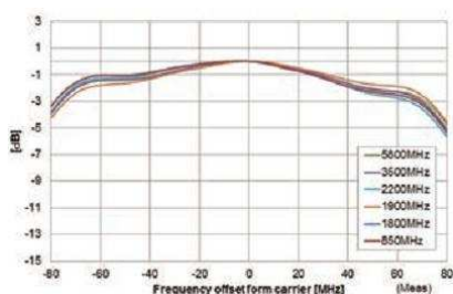
График полосы пропускания I/Q с использованием опционального внутреннего генератора основной полосы
