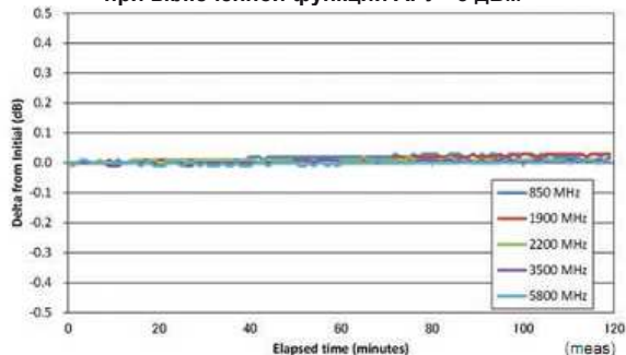
Дрейф
