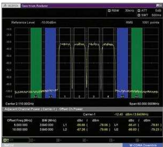
W-CDMA ACLR, 4 несущих (TestModel1, 64DPCH, 4 несущих)
