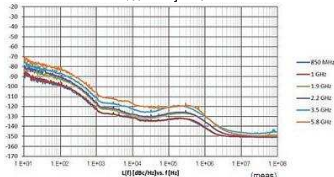
Фазовый шум в ОБП
