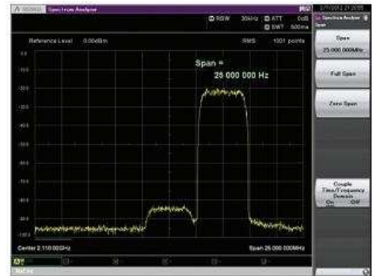
Спектр комбинации «полезный сигнал + модулированный сигнал помехи»
