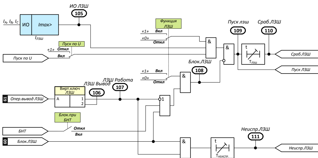
Рисунок 11 – Функционально-логическая схема ЛЗШ
