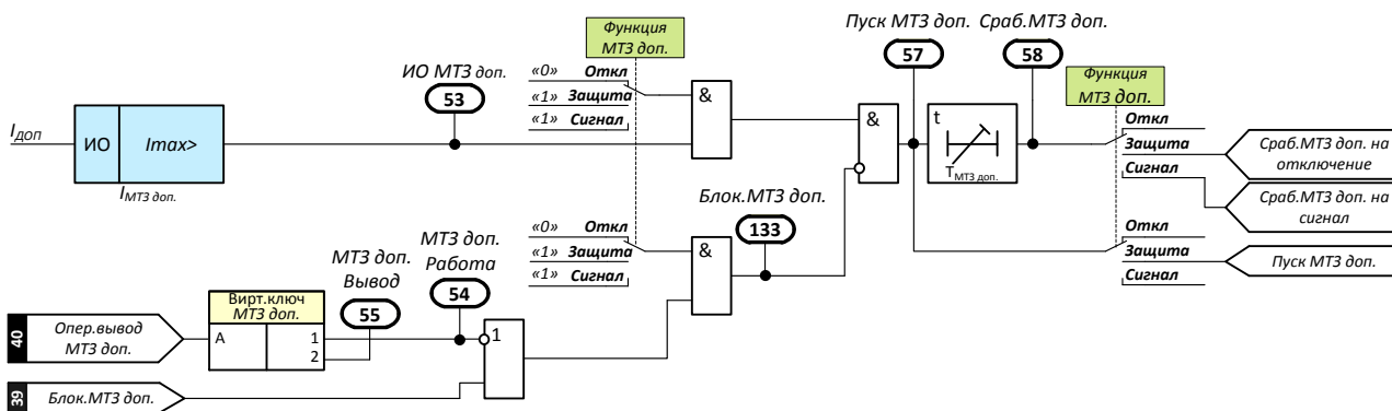
Рисунок 10 – Функционально-логическая схема МТЗ-доп.
