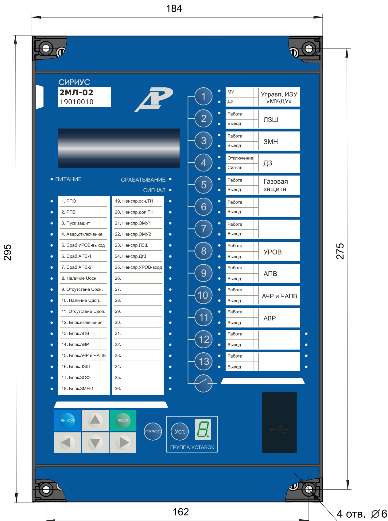
Рисунок А.1 – Вид спереди (лицевая панель LA41) для исполнений K450-41 и K401-41
