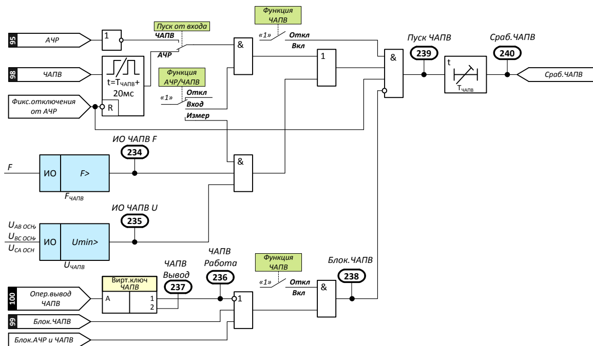
Рисунок 36 – Функционально-логическая схема частотного автоматического повторного включения
