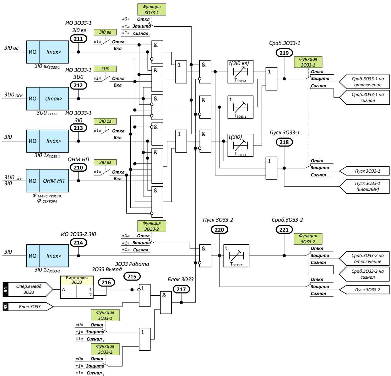
Рисунок 16 – Функционально-логическая схема 3033
