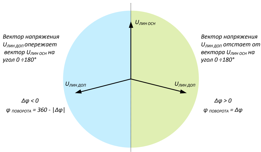
Рисунок 52 – Поясняющая диаграмма определения значения уставки «φ поворота»
