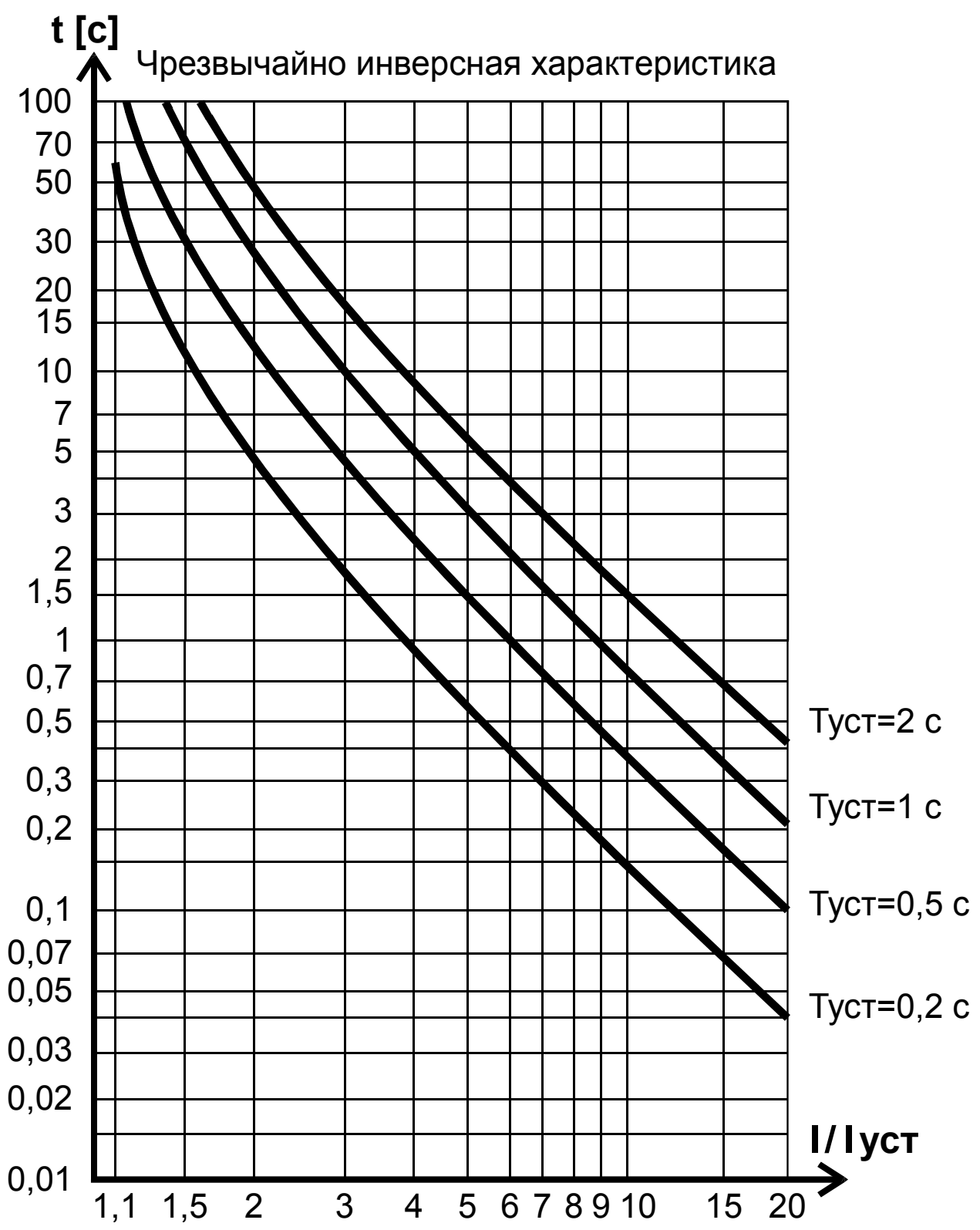
Рисунок М.3 – Чрезвычайно инверсная характеристика по МЭК 255-4
