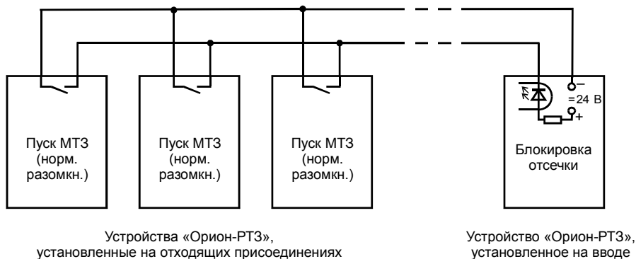
Рисунок 3 – Схема соединения нескольких устройств «Орион-РТЗ» между собой при организации логической защиты шин (параллельная схема)
