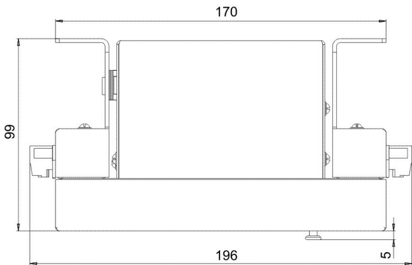
Рисунок 10в – Вид на устройство сверху (переднее присоединение)
