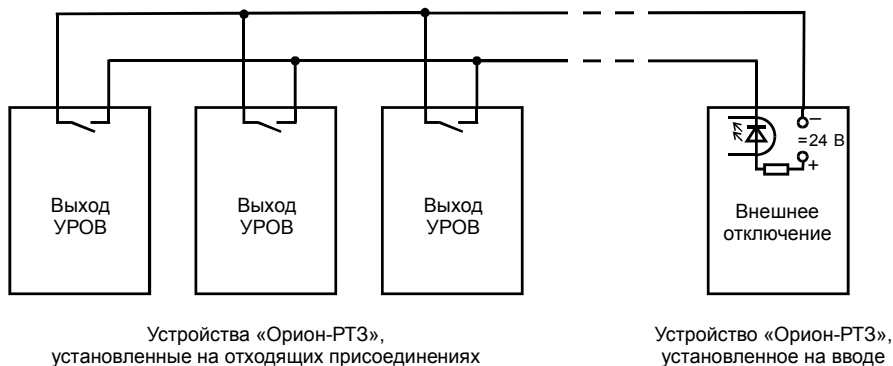
Рисунок 2 – Схема соединения нескольких устройств «Орион-РТЗ» между собой для реализации УРОВ на подстанции
