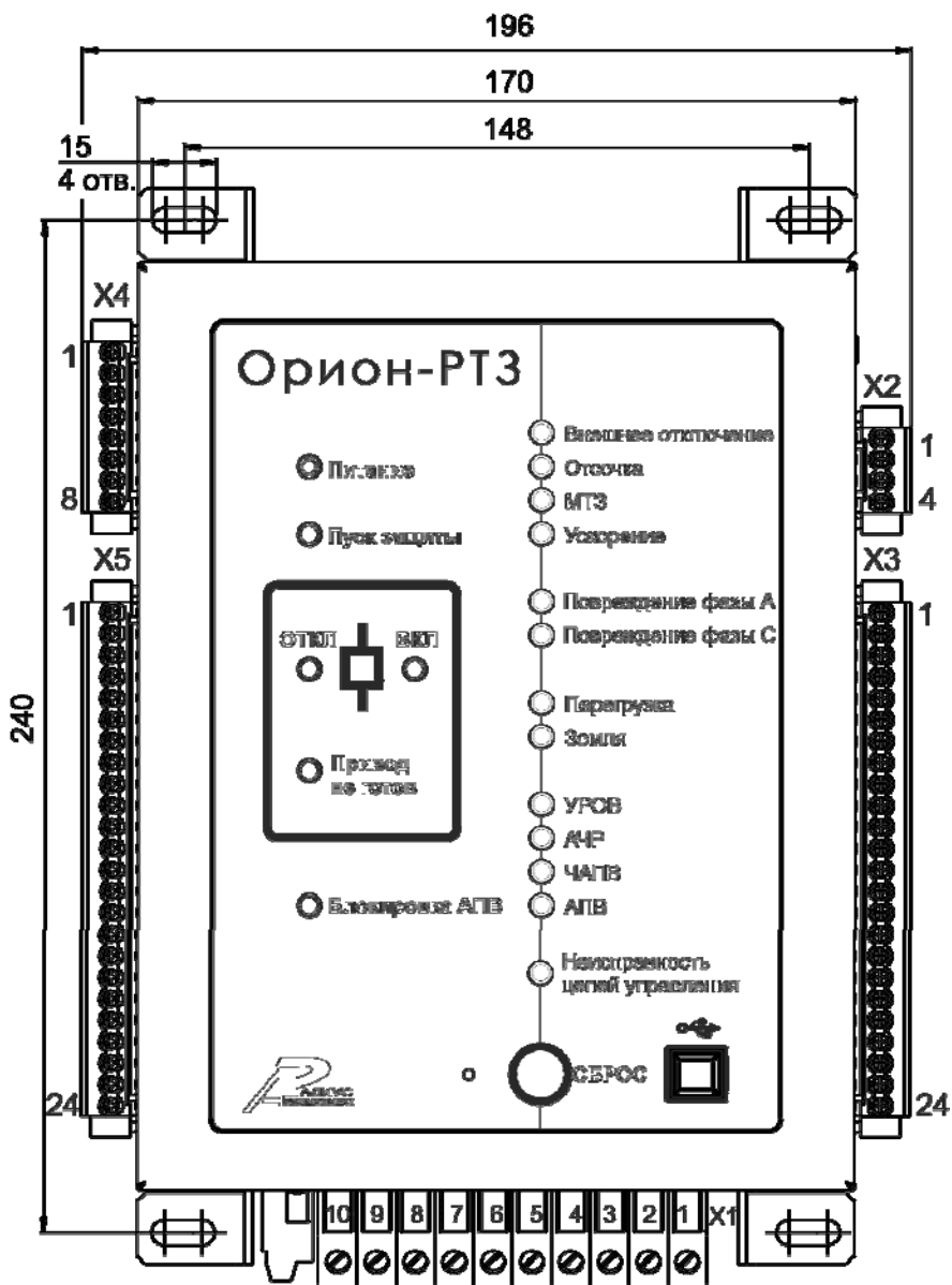
Рисунок 86 – Вид передней панели устройства (переднее присоединение)
