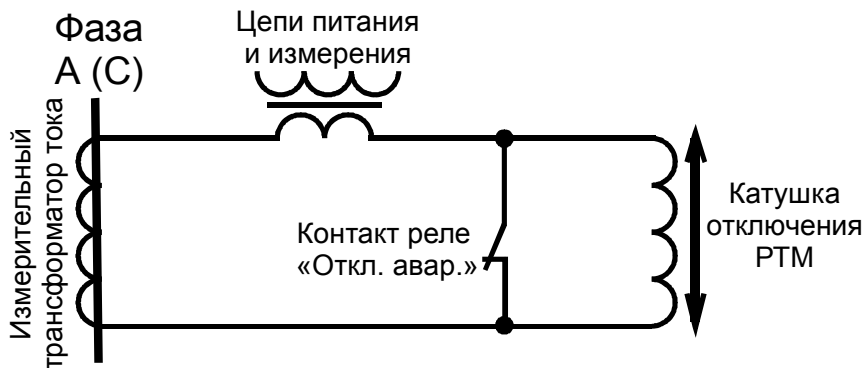
Рисунок 1 – Схема организации токовой цепи каждой из фаз А и С при применении схемы дешунтирования для аварийного отключения выключателя
