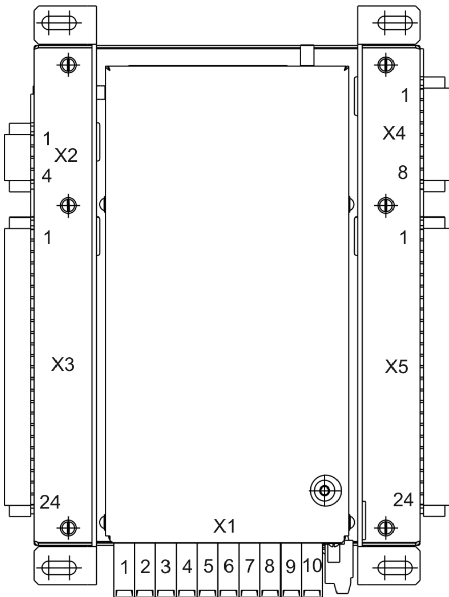
Рисунок 11б – Вид сзади (переднее присоединение)
