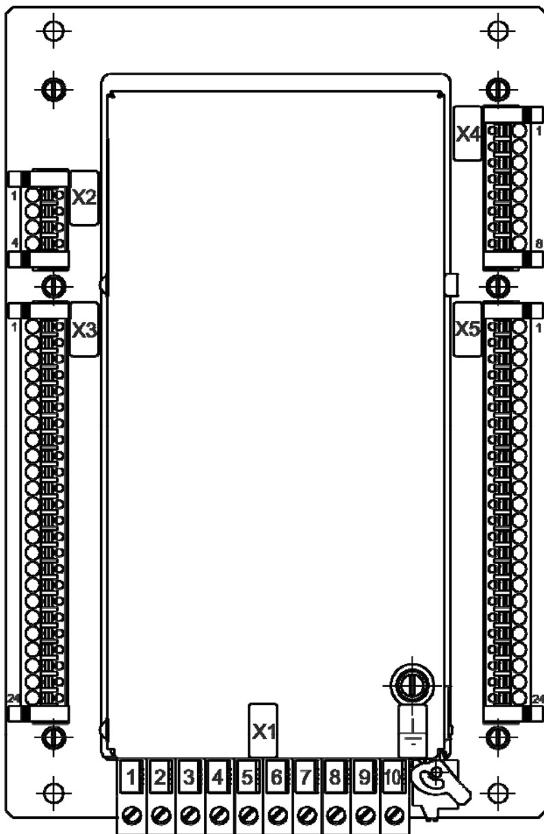
Рисунок 11а – Вид сзади со стороны клемм подключения (заднее присоединение)
