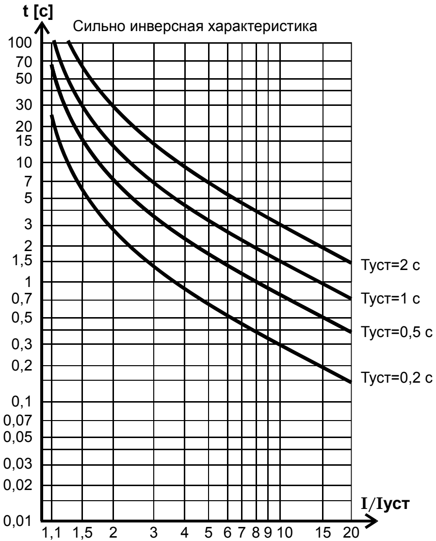
Рисунок 14 – Сильно инверсная характеристика по МЭК 255-4
