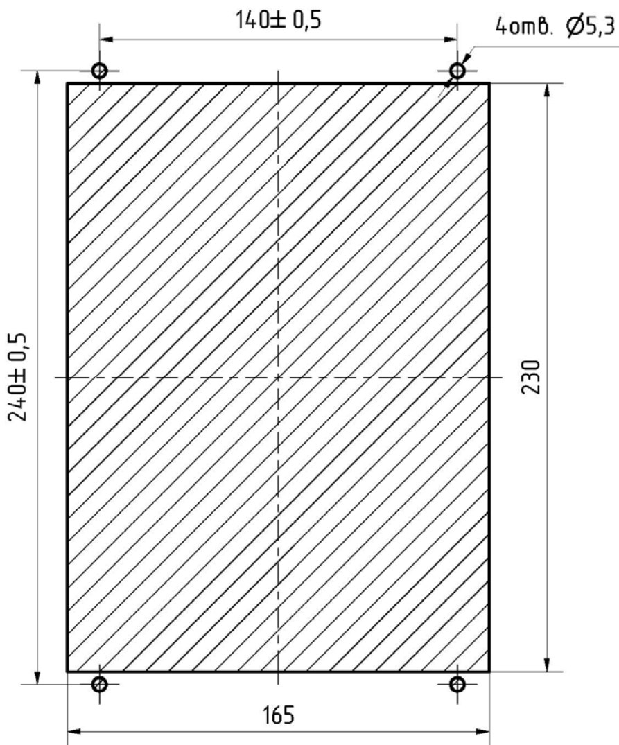
Рисунок 12 – Вырубаемое окно в панели (для заднего присоединения)
