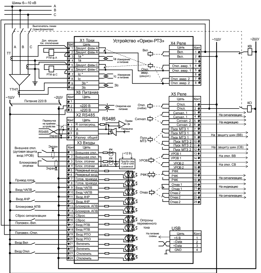
Рисунок 6 – Схема подключения устройства «Орион-РТЗ» к выключателю по схеме дешунтирования
