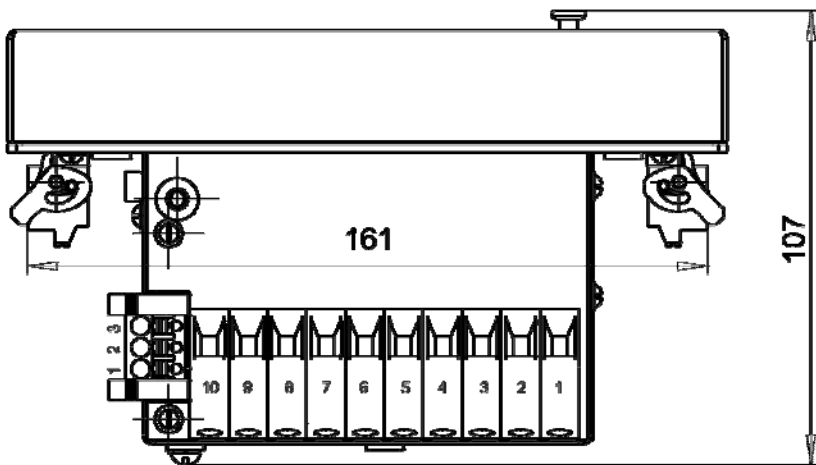
Рисунок 10б – Вид на устройство снизу (заднее присоединение)
