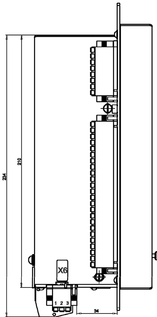
Рисунок 9а – Вид на устройство сбоку (заднее присоединение)
