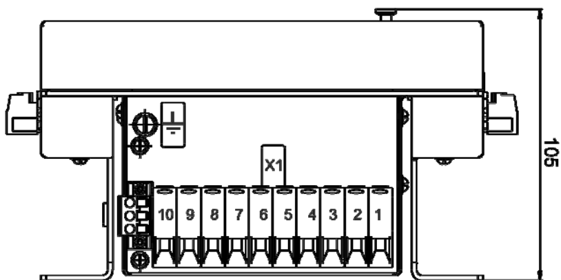
Рисунок 10г – Вид на устройство снизу (переднее присоединение)
