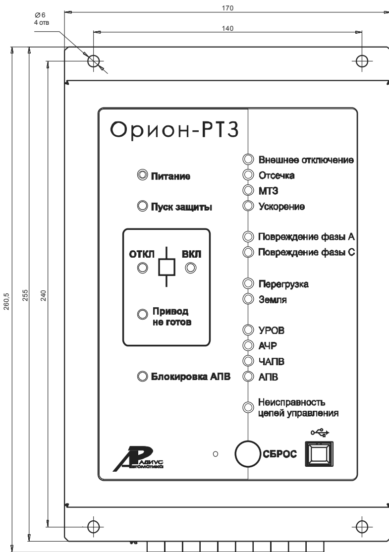
Рисунок 8а – Вид передней панели устройства (заднее присоединение)
