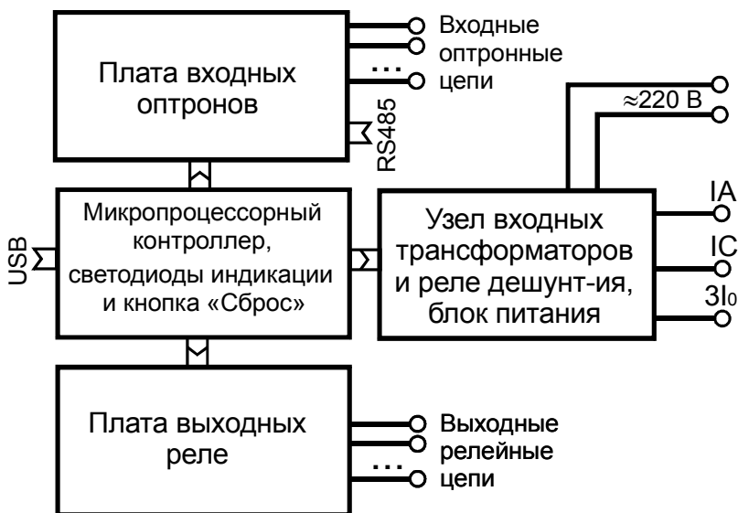
Рисунок 4 – Структурная схема устройства «Орион-РТЗ»
