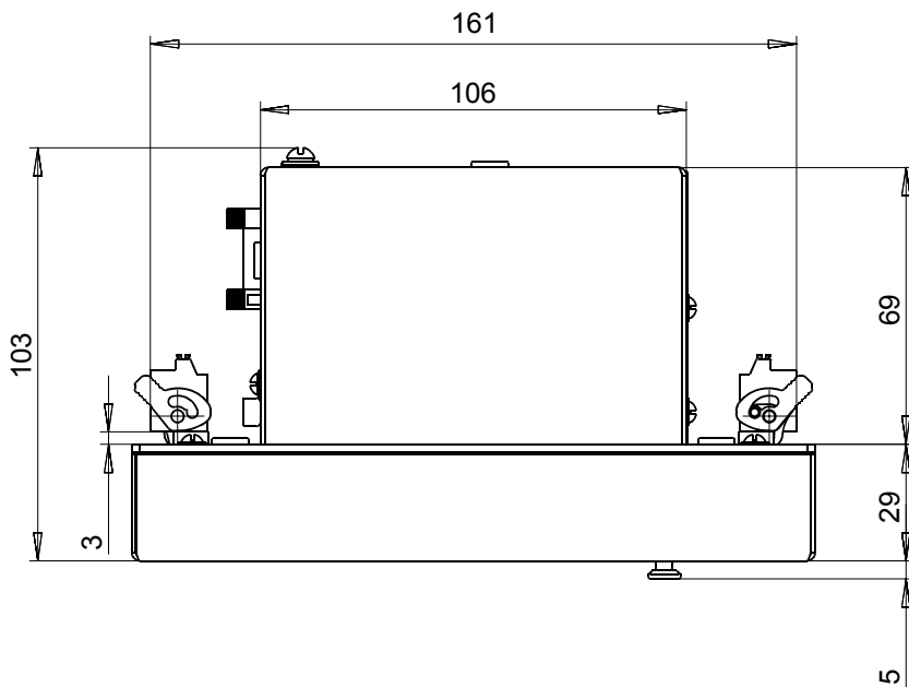
Рисунок 10а – Вид на устройство сверху (заднее присоединение)
