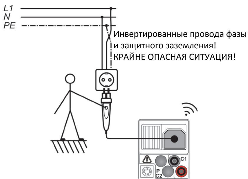
Рисунок 5.43: Инвертированные провода фазы и защитного заземления (L и PE) (щуп типа командер с вилкой (plug commander))
