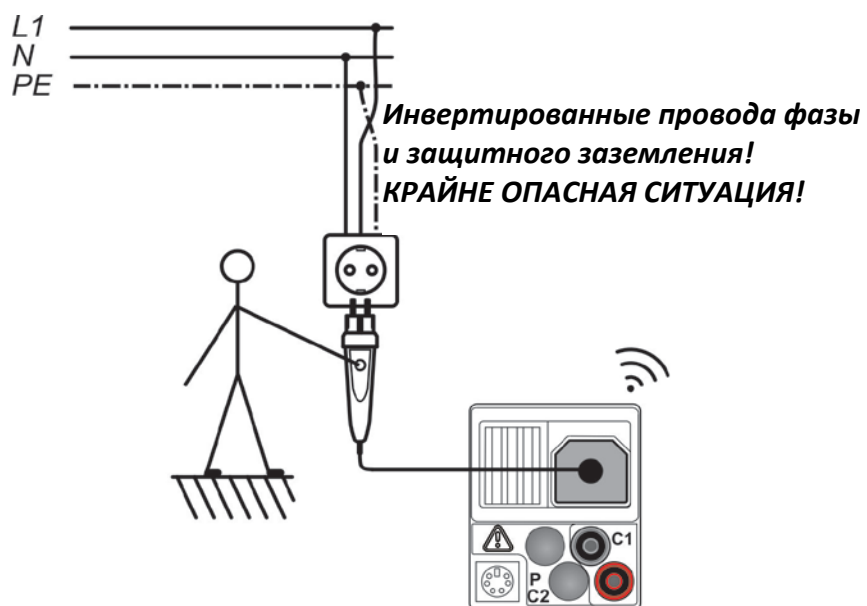
Рисунок С.4: Инвертированные проводники L и PE (применение щупа «plug commander»)
