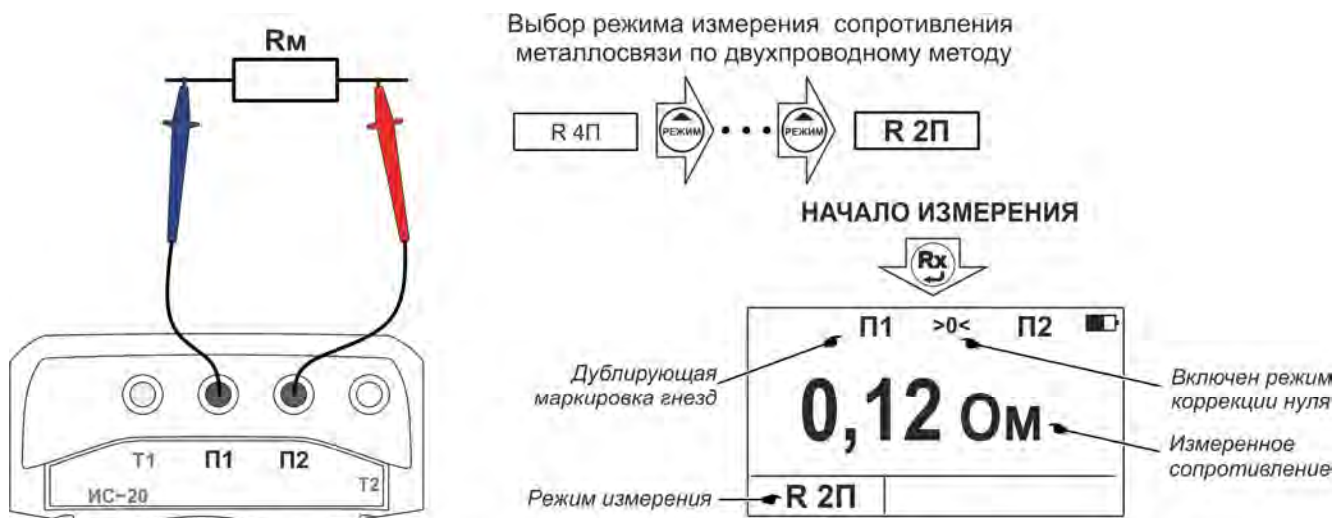
Рисунок 2.8 – Схема подключения и вид индикатора
