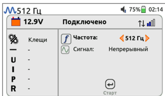
Рисунок 6.5 Параметры генератора при работе с индукционными клещами.
