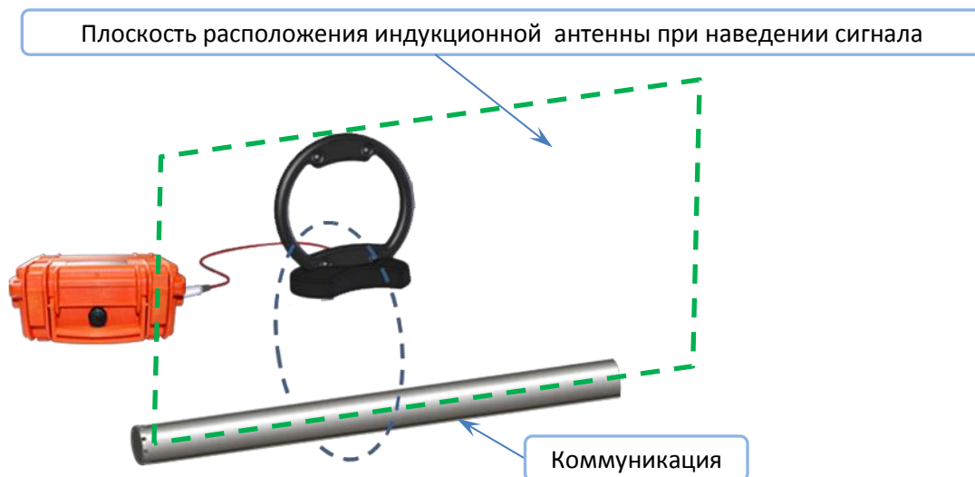
Рисунок Г.1 Наведение сигнала индукционной антенной ИЭМ-301.X
