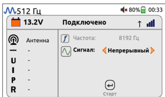
Рисунок 6.6 Выбор параметров генератора при работе на внешнюю антенну.
