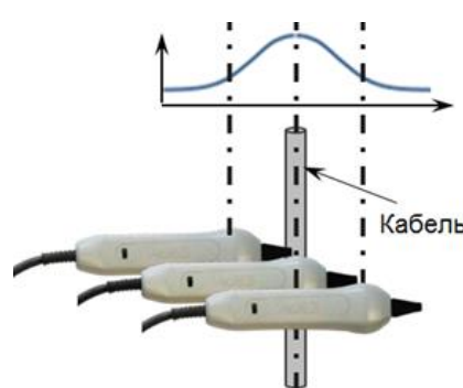
Рисунок А.2 Оси чувствительности датчика MED-127.
