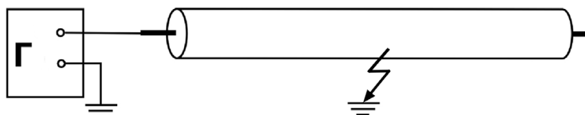
Рисунок В.6 Схема подключения генератора при поиске дефектов изоляции.
