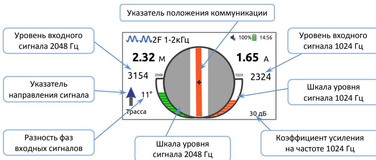
Рисунок 3.16. Режим «Трасса» при двухчастотном режиме.
