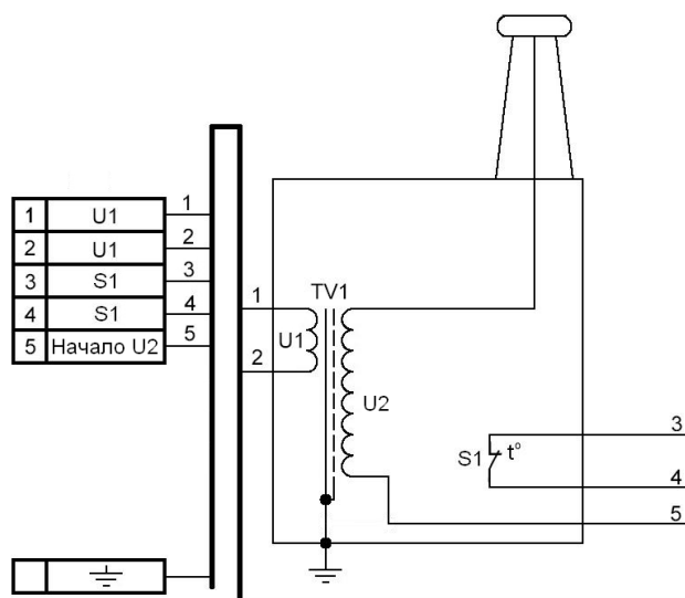
Рис 1. Трансформатор ТВИ-100/100.
