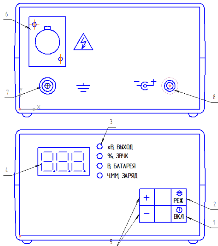
Рис.2. Панели блока контроля
