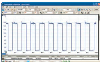
КЛАПАН ХОЛОСТОГО ХОДА
