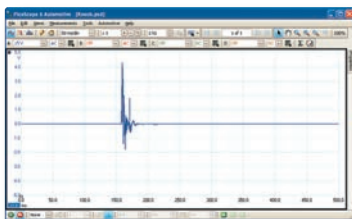
ДАТЧИК ДЕТОНАЦИИ
