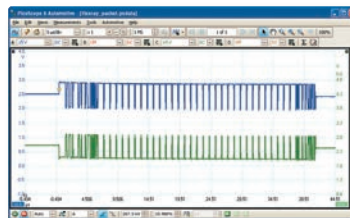
ШИНА FLEXRAY
