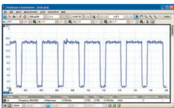
EGR КЛАПАН
