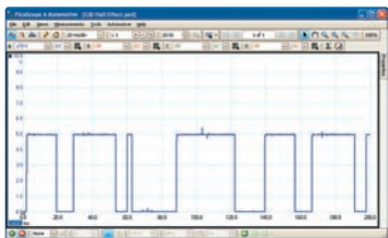
ДАТЧИК ХОЛЛА
