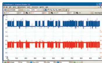
ШИНА CAN
